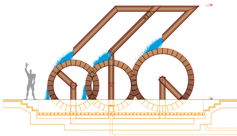
Plan technique de la fontaine du Millénaire, réalisé par Mario Botta
